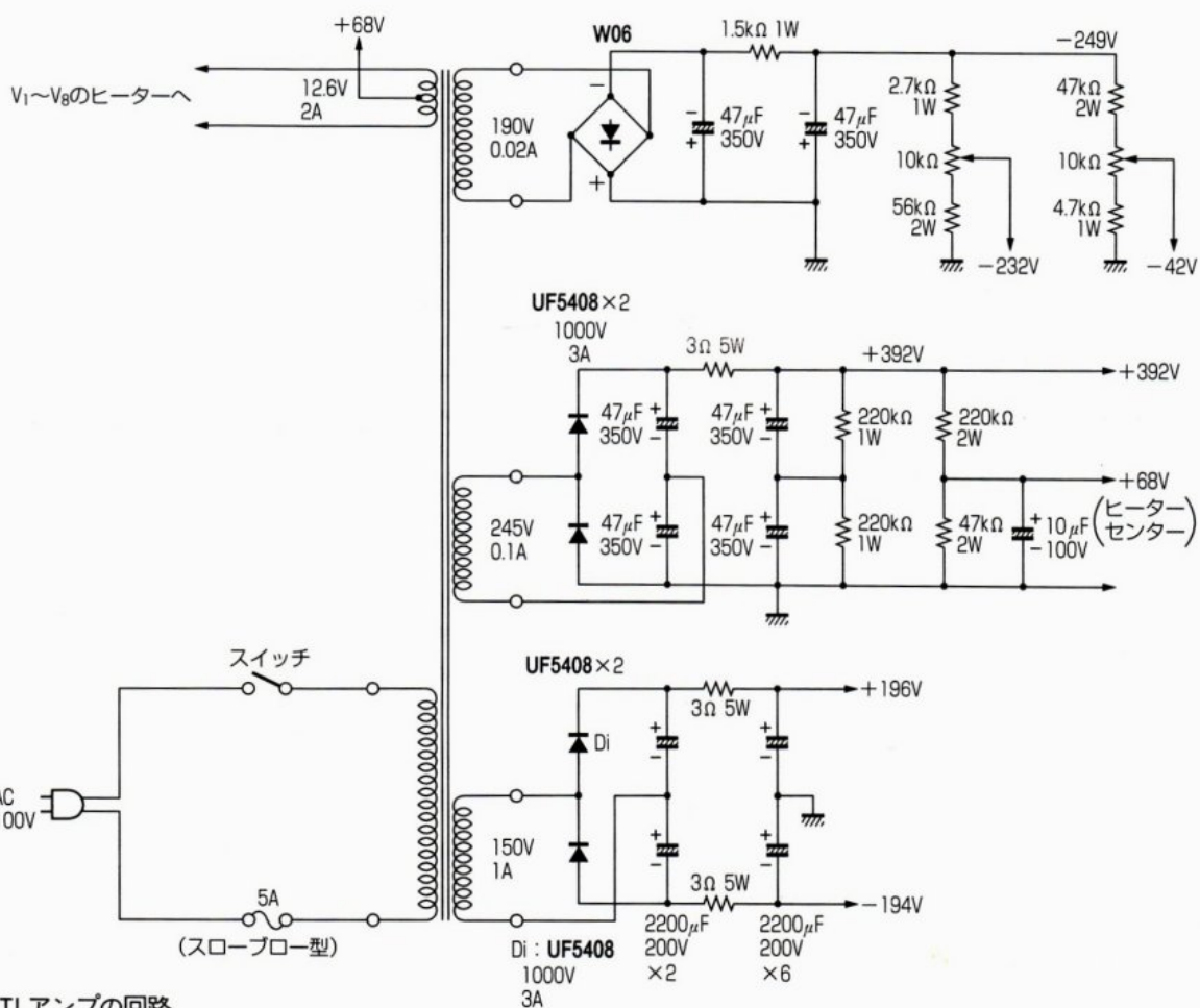
【図7】 改造型II型OTLアンプの回路
