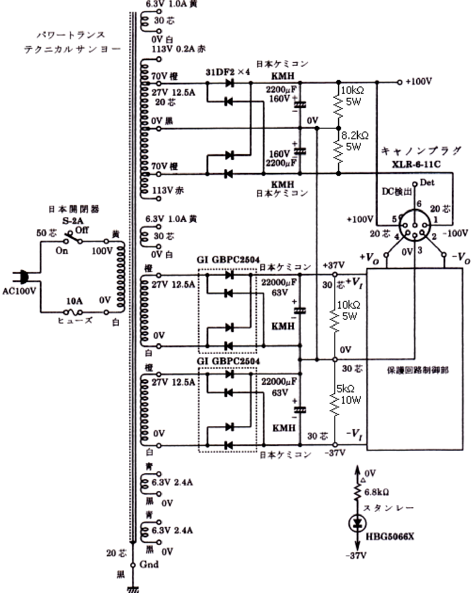
【図2】 電源部回路
